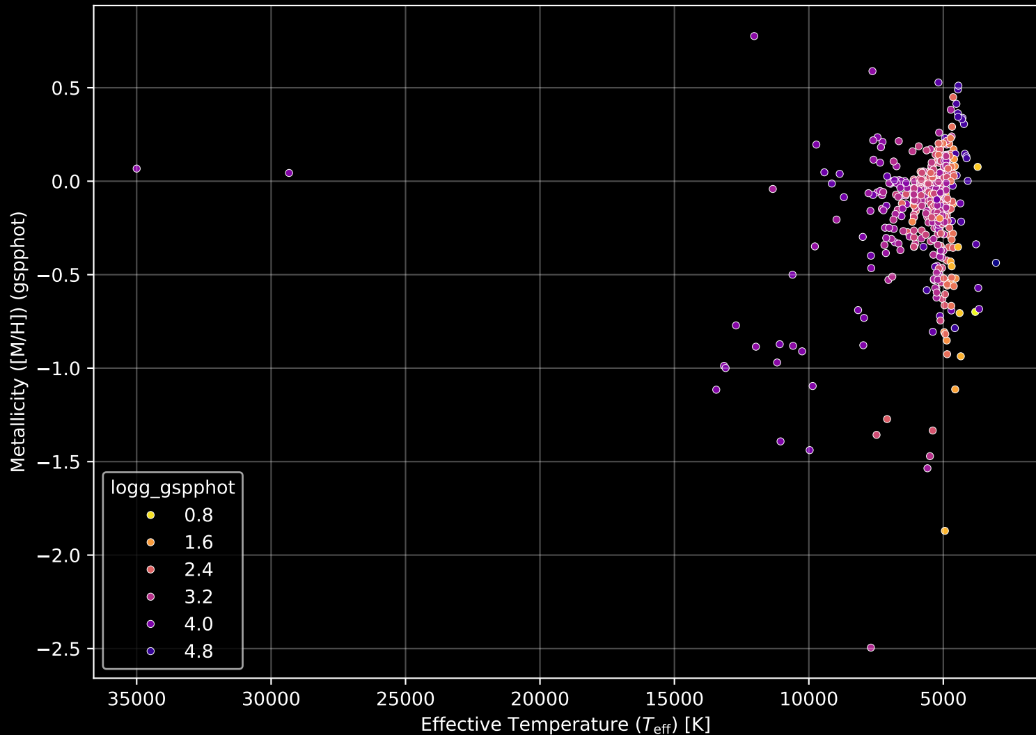
APOGEE DR17 Field: [195+00] Stellar Population Parameters (n= 495)
